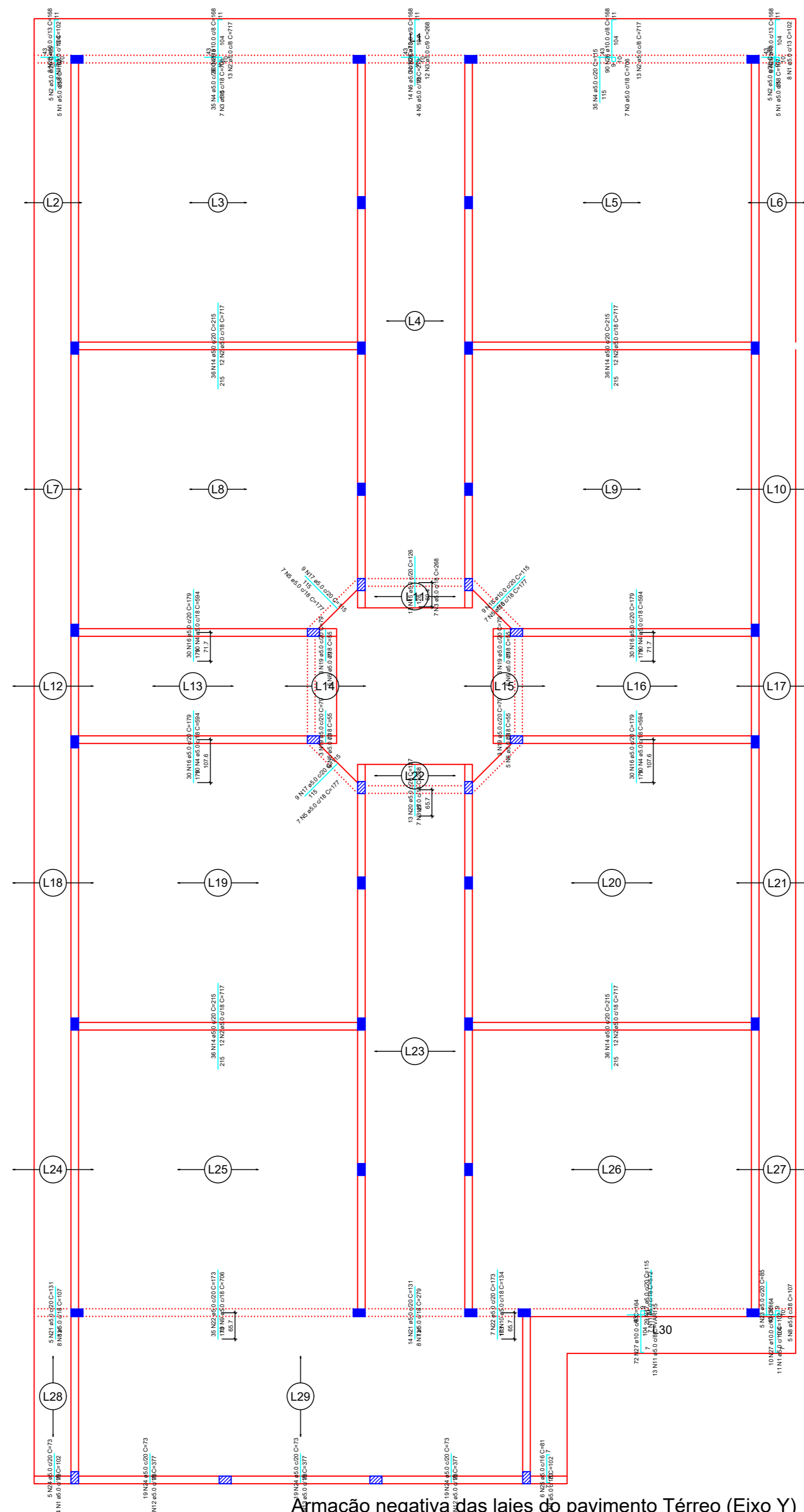
Armação negativa das lajes do pavimento Térreo (Eixo Y) escala 1:50
