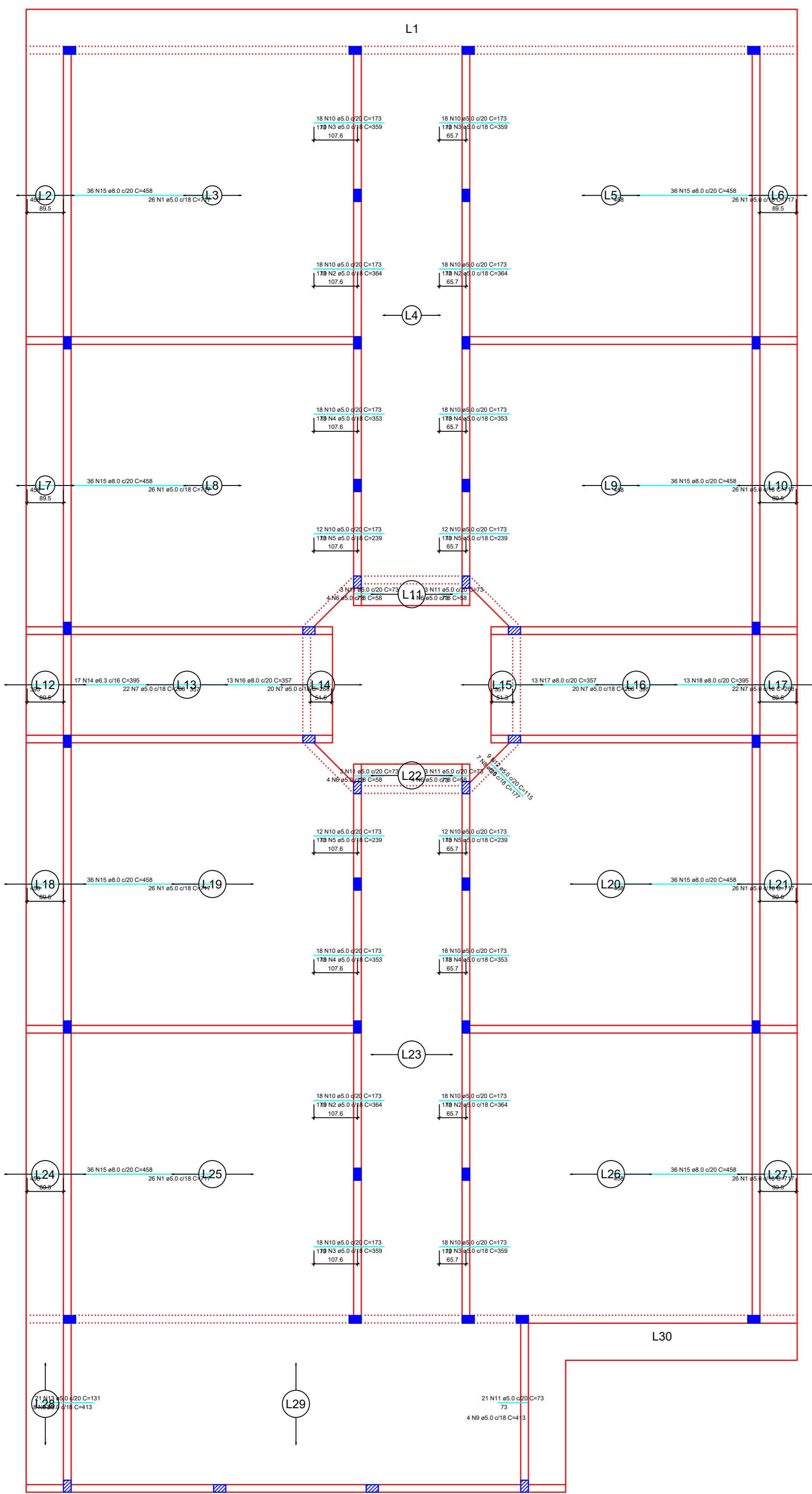
Armação negativa das lajes do pavimento Térreo (Eixo X) escala 1:50
